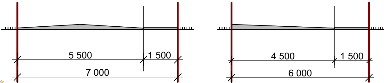
СХЕМА ПОПЕРЕЧНИХ ПРОФІЛІВ ВУЛИЦЬ ТА ДОРІГ
